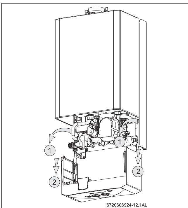
Fig. 11 Position de service
