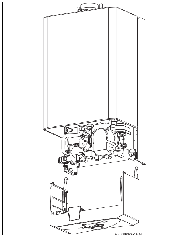
Fig. 12 Enlever le tableau électrique
