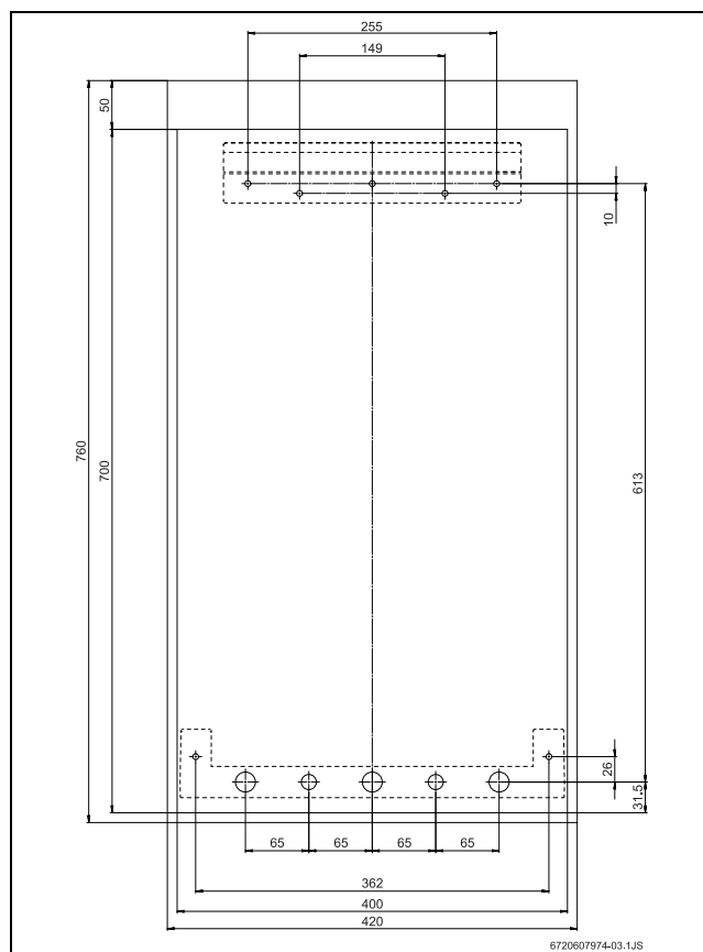
Fig. 9 Montage de la traverse d'accrochage et de la plaque de pré-installation
