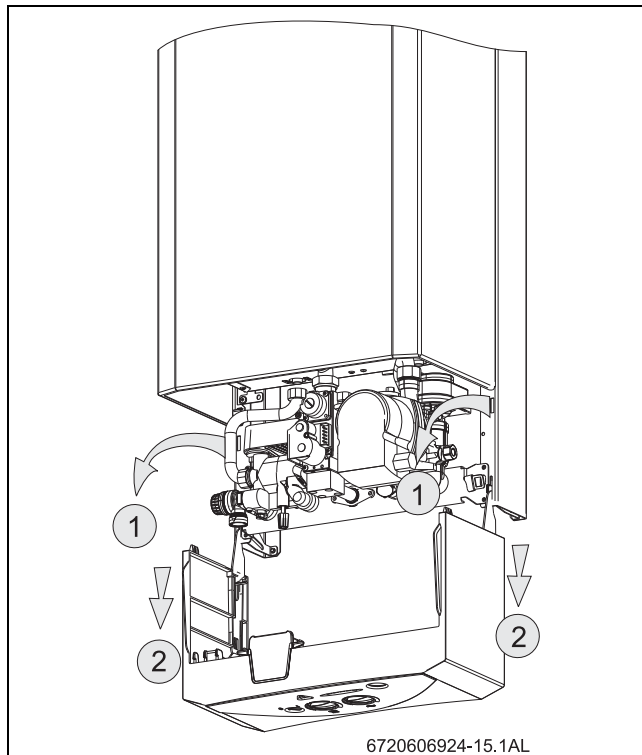
Fig. 29 Position de réglage pour accéder à l'électronique et de l'hydraulique
