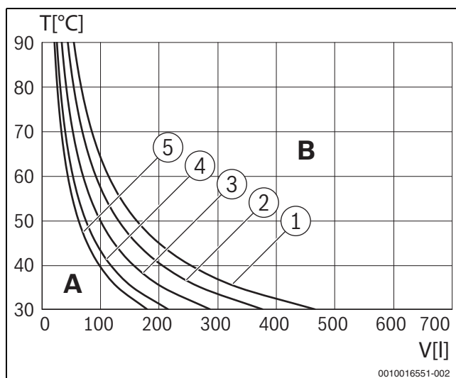
Fig. 7 Courbes caractéristiques du vase d'expansion
