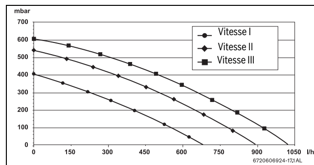
Fig. 6 Caractéristique du circulateur
