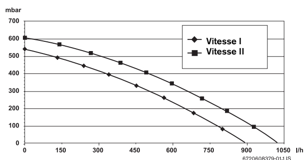
Fig. 6 Caractéristique du circulateur
