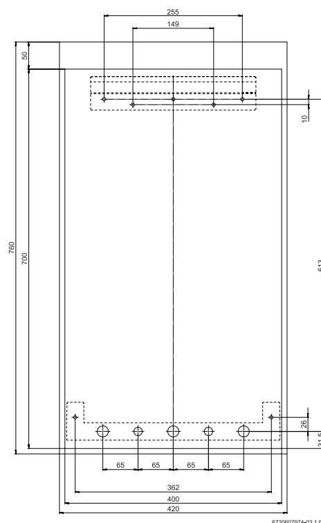
Fig. 8 Montage de la traverse d'accrochage et de la plaque de pré-installation
