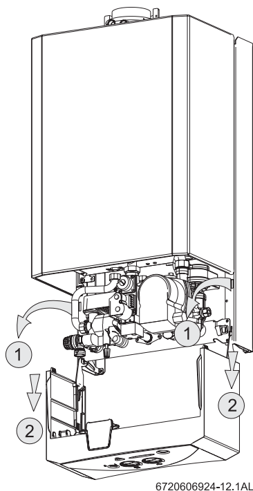
Fig. 10 Position de service
