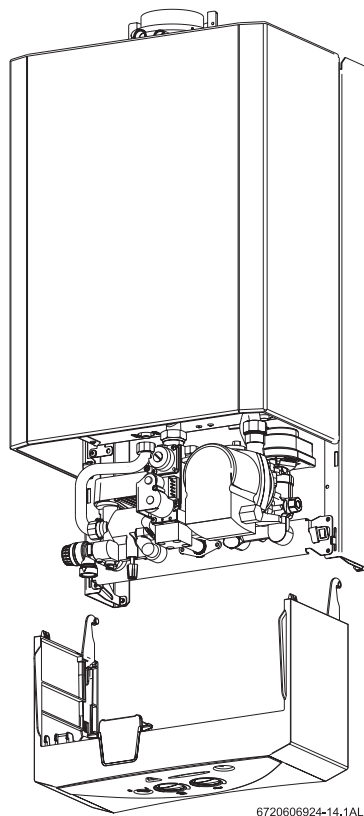
Fig. 11 Enlever le tableau électrique
