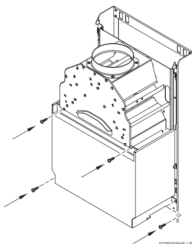
Fig. 26 Couvercle de protection
