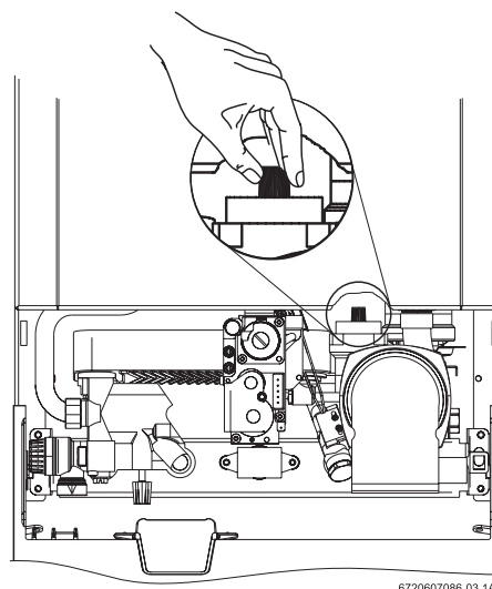
Fig. 13 Ouvrir la valve de purge
