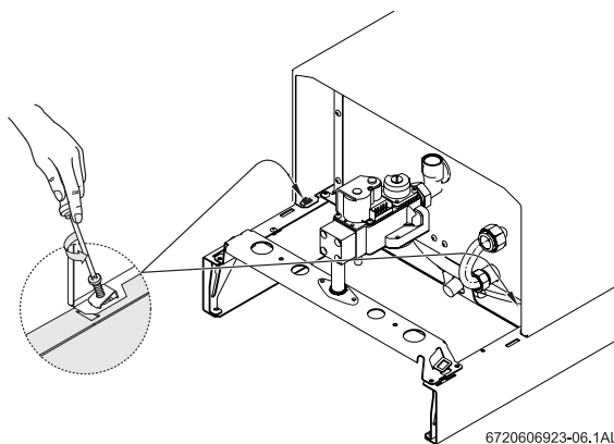
Fig. 12 Habillage
