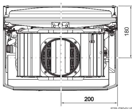
Fig. 2 Vue de dessus
