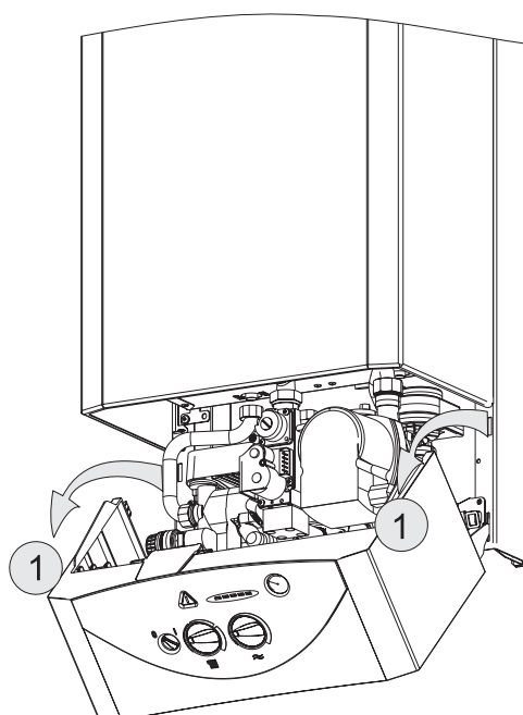
Fig. 24 Position de réglage
