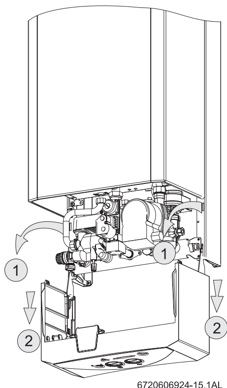
Fig. 28 Position de réglage pour accéder à l'électronique et de l'hydraulique
