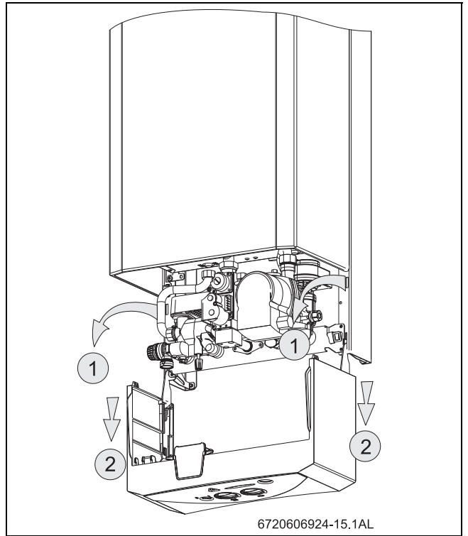
Fig. 26 Position de réglage pour accéder à l'électronique et de l'hydraulique
