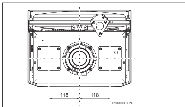
Fig. 2 Vue de dessus
