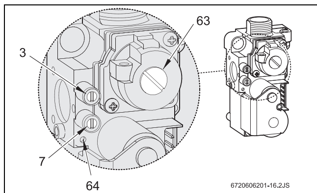
Fig. 23 Bloc de gaz
