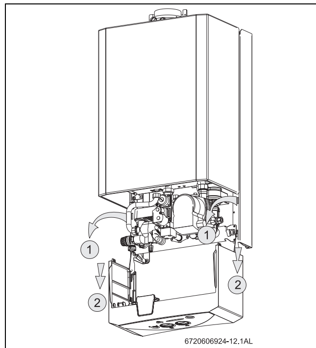
Fig. 9 Position de service
