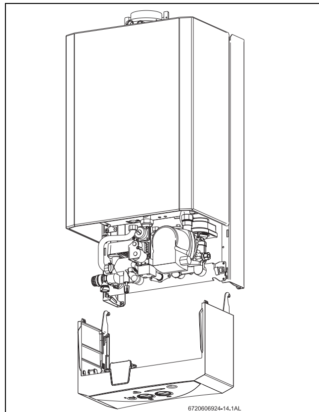
Fig. 10 Enlever le tableau électrique
